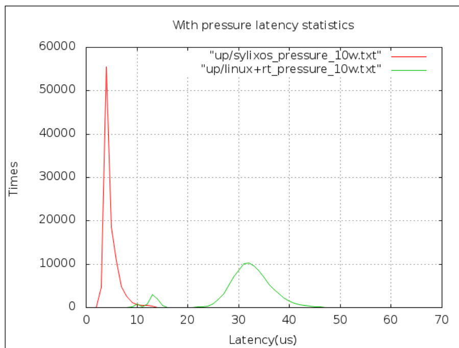
图 3.12 SylixOS、Linux+RT 单核 10w 有压力延迟次数统计
