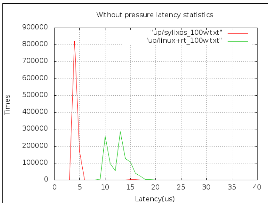
图 3.11 SylixOS、Linux+RT 单核 100w 无压力次延迟次数统计
